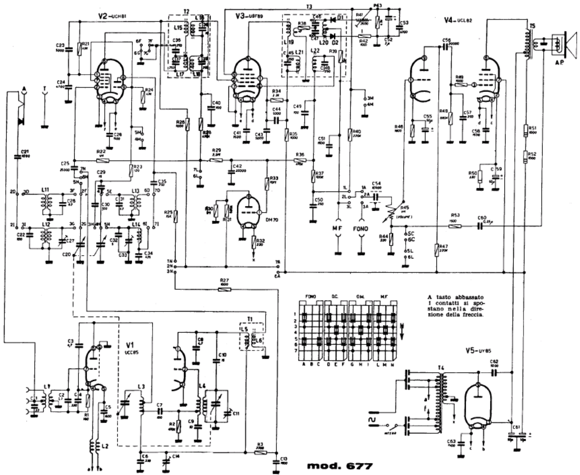
Mod. 677. Apparecchio a modulazione d'ampiezza e di frequenza. Gamma onde medie da 520 a 1620 kc/s.
